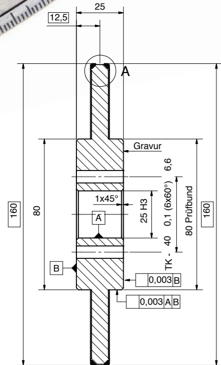
CVD-Abrichtrolle
